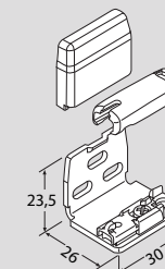
Zijgeleidsbeugel voor achterzijde montage (optioneel) Type A011
