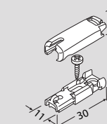
Zijgeleidsbeugel voor onderzijde montage (optioneel) Type A011
